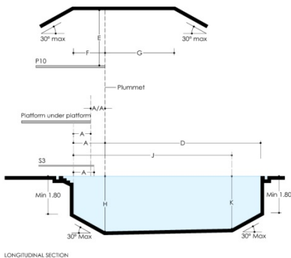
LONGITUDINAL SECTION
